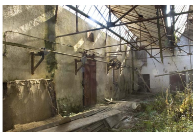
Atelier de fabrication. Charpente métallique et éléments de transmission. Phot. Jérôme Mongreville IVR43_20097000281NUC2A
