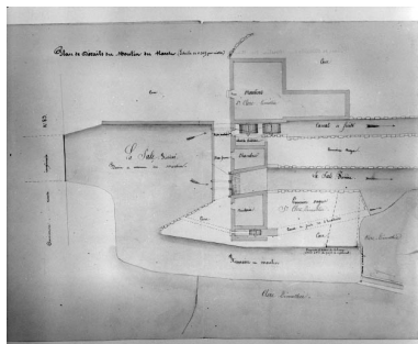
Plan et dessins de détail. Réglementation de l'usine dite moulin du Haut [...]. Phot. Jérôme Mongreville, Autr. Charpy IVR43_19963900200X
