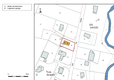
Plan-masse et de situation. Extrait du plan cadastral, 2017, section ZD, 1/1 000. Dess. Mathias Papigny IVR43_20172501301NUDA
