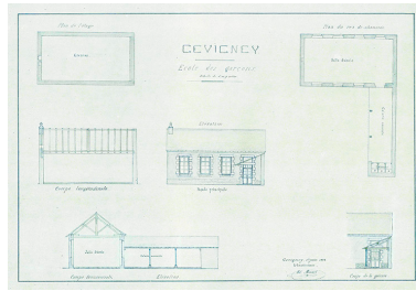
Plan de l'école réalisé en 1888. Autr. auteur inconnu IVR43_20177000003NUC4A
