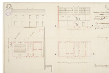
Projet d'aménagement de l'école par l'architecte Renahy (1843). Phot. Jérôme Mongreville, Autr. Adrien Renahy IVR43_20167000970NUC4A
