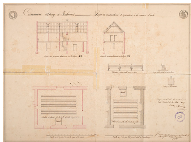
Projet d'aménagement de l'école par l'architecte Renahy (1843). Phot. Jérôme Mongreville, Autr. Adrien Renahy IVR43_20167000968NUC4A
