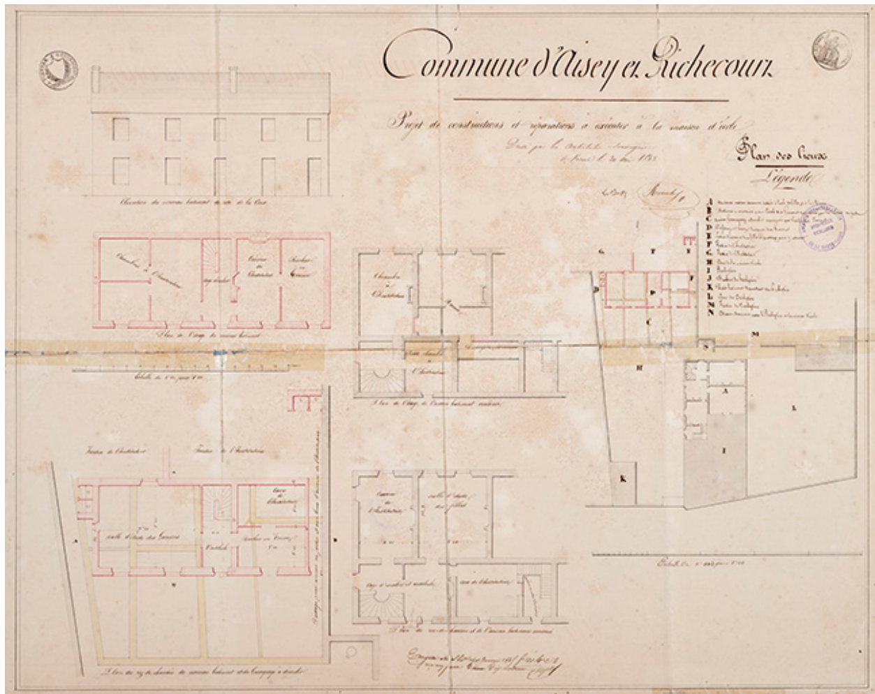
Projet d'aménagement de l'école par l'architecte Renahy (1843).
