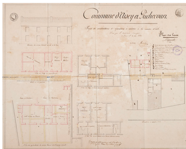
Projet d'aménagement de l'école par l'architecte Renahy (1843). Phot. Jérôme Mongreville, Autr. Adrien Renahy IVR43_20167000969NUC4A
