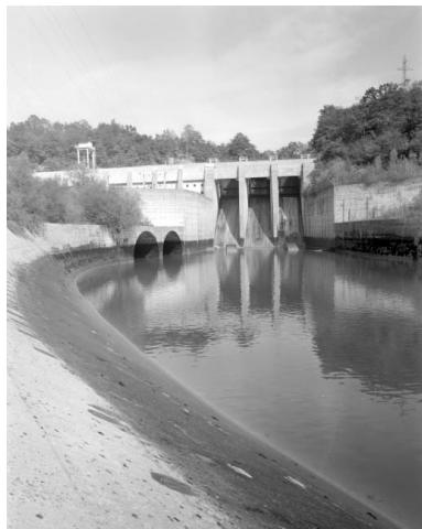
Evacuateur et bassin d'amortissement (cadrage vertical). Phot. Jérôme Mongreville IVR43_19913900651X
