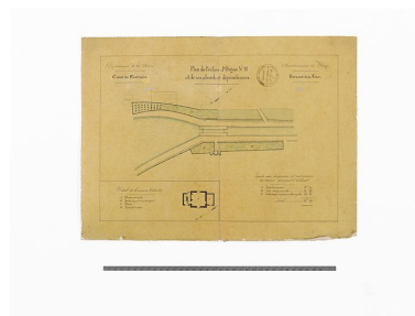
"Plan de l'écluse d'Orgue n°11 et de ses abords et dépendances". Plan général du site d'écluse et détail de la maison éclusière. (Plan aquarellé ; 41,5 x 30,5 cm, Archives VNF-direction territoriale Centre-Bourgogne ; subdivision de Corbigny) Phot. Thierry Kuntz IVR26_20135800018NUC4A
