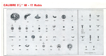
Calibre 5 1/2''' 68 - 17 rubis [éclaté des fournitures], 1973. Autr. auteur inconnu IVR43_20162500104NUC4A
